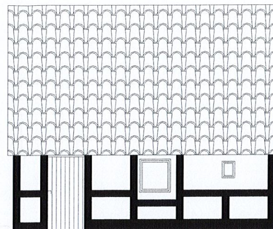
Elewacja północno-wschodnia
