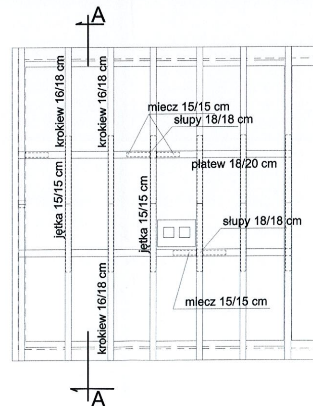
Rzut więźby dachowej
