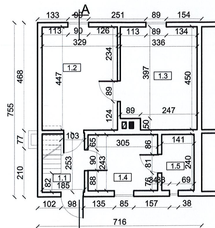
Rzut parteru
