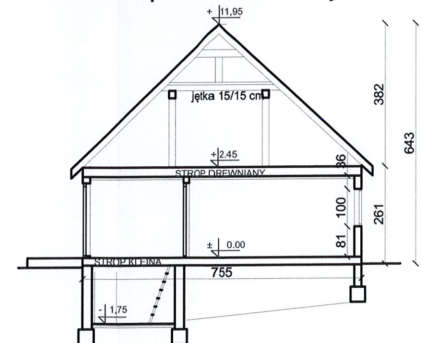
Przekrój A - A
