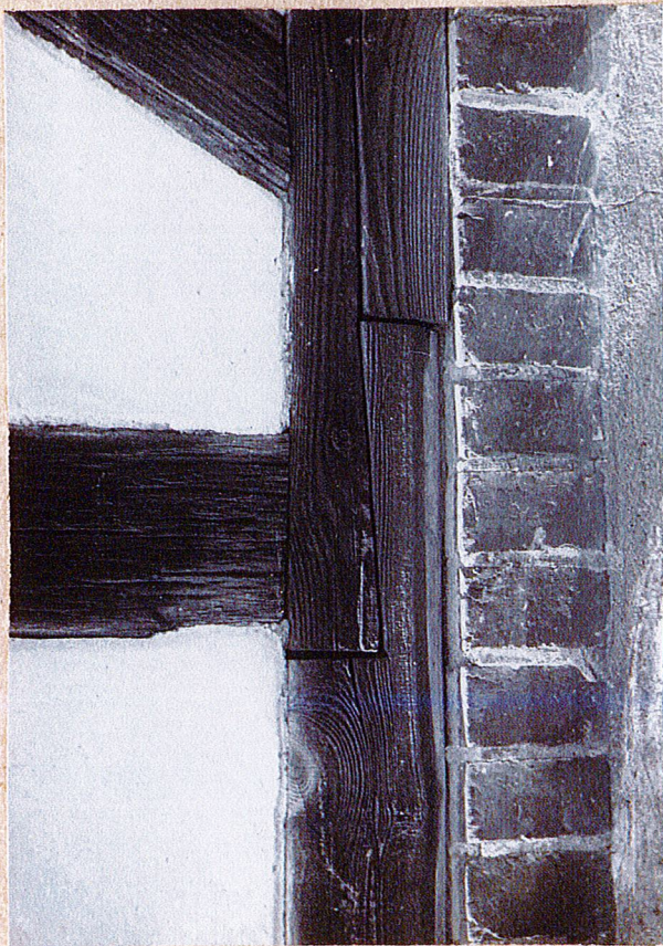
Elewacja pld., łączenie ciesielskie.
