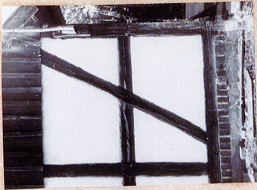
Elewacja pld., fragment konstrukcji.
