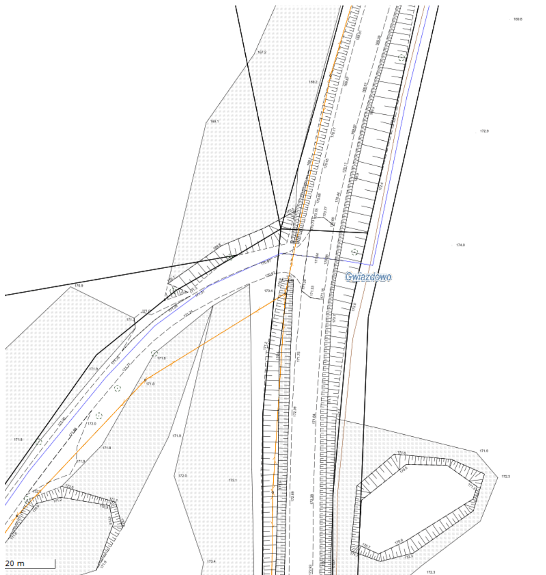
Mapa zasadnicza- droga wojewódzka DW 171 i włączenie do istniejącej sieci kanalizacji sanitarnej na działce ewidencyjnej 49/14
