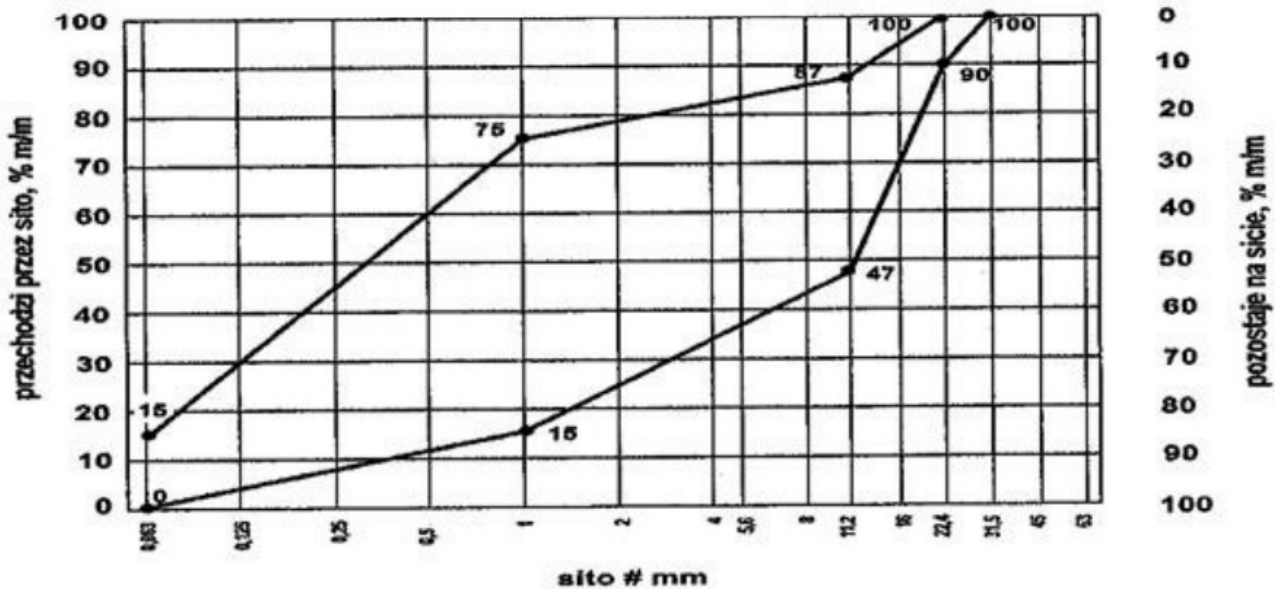
Rys. 3. Krzywe graniczne uziarnienia mieszanki kruszyw 0/16 mm do górnej warstwy podłoża ulepszanego
