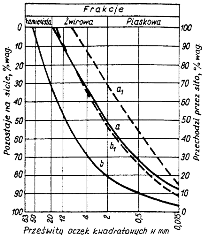
Rysunek 1. Obszar uziarnienia optymalnych mieszanki żwirowych
