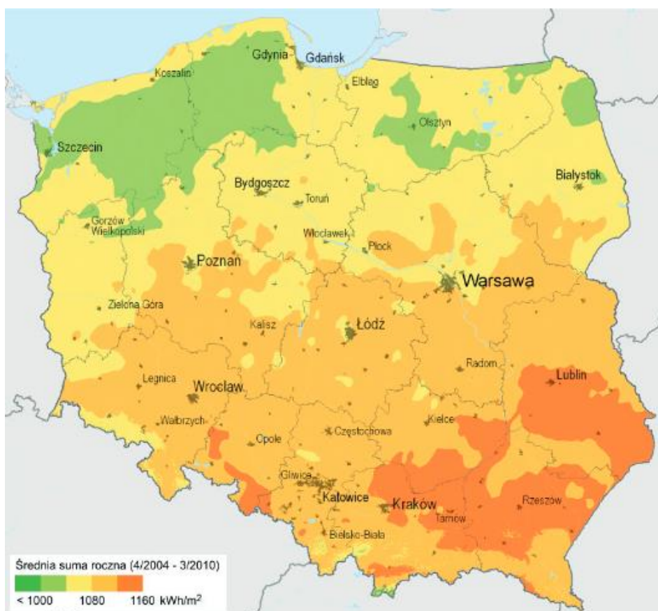
Ryc. 20. Rozkład rocznych wartości nasłonecznienia w Polsce
