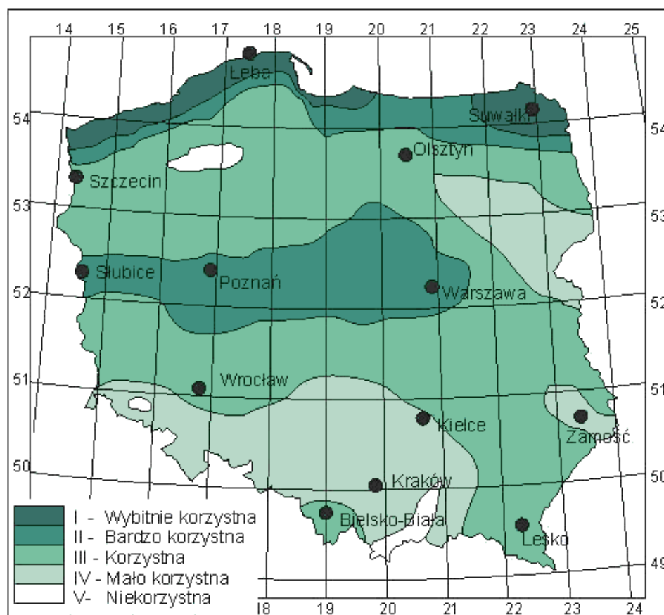
Ryc. 19. Strefy energetyczne wiatru w Polsce
