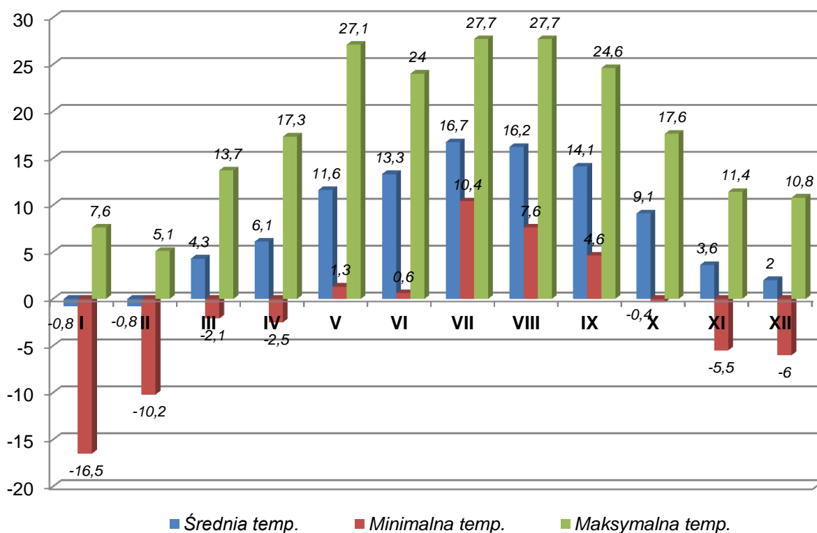
Wykres 2. Średnia, minimalna i maksymalna temperatura poszczególnych miesięcy dla typowego roku meteorologicznego dla stacji meteorologicznej w Koszalinie
