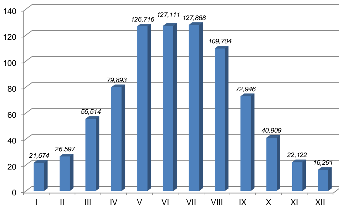
Wykres 40. Natężenie promieniowania słonecznego na powierzchnię poziomą dla typowego roku meteorologicznego dla stacji meteorologicznej w Koszalinie [kWh/m 2 ]
