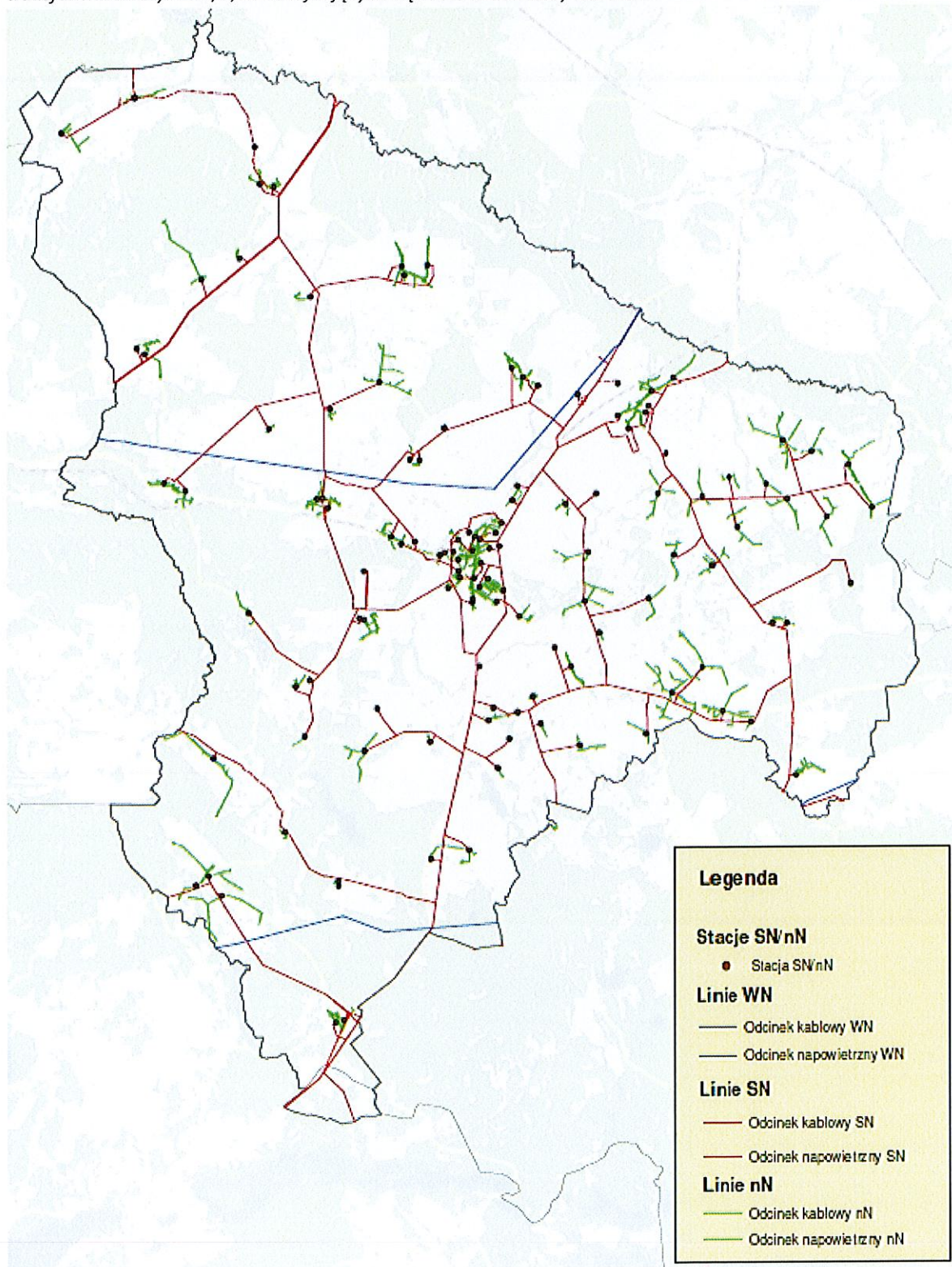
Rysunek 3. Aktualny plan rozmieszczenia sieci elektroenergetycznych 110 kV, 15 kV i 0,4 kV oraz stacji transformatorowych 15/0,4kV znajdujących się na terenie Gminy Barwice
